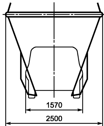
Рисунок 2 - Выступание наружных элементов траверс за контуры груза при необходимости обеспечения его сохранности
