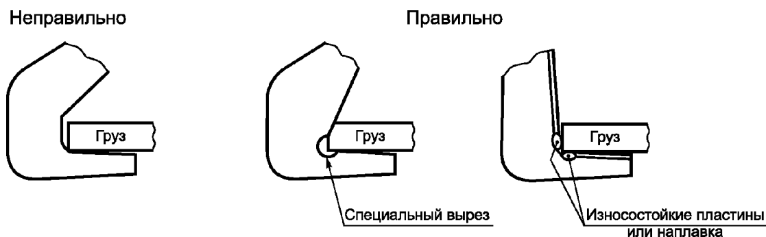
Рисунок 4 - Конструкция захватов ГЗП
