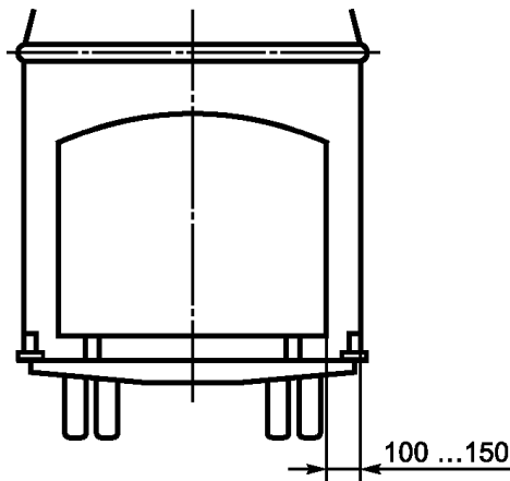
Рисунок 1 - Выступание наружных элементов траверс за контуры груза
