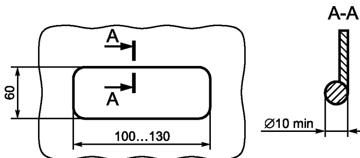
Рисунок 7 - Рекомендуемые размеры отверстий для хвата рукой
