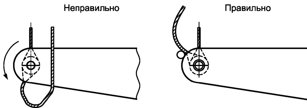
Рисунок 8 - Устройства, исключающие образование петель и перекруток
