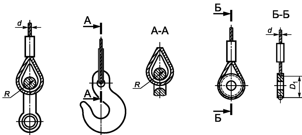
Рисунок 5 - Петли канатных ветвей, входящих в состав ГЗП
