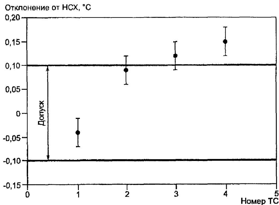
Рисунок В.1. Условия приемки и отбраковки ТС класса АА по результатам измерений при 0 °С. Из четырех показанных ТС только ТС N 1 может быть принят изготовителем (или поверочным центром) и только ТС N 4 может быть забракован потребителем
