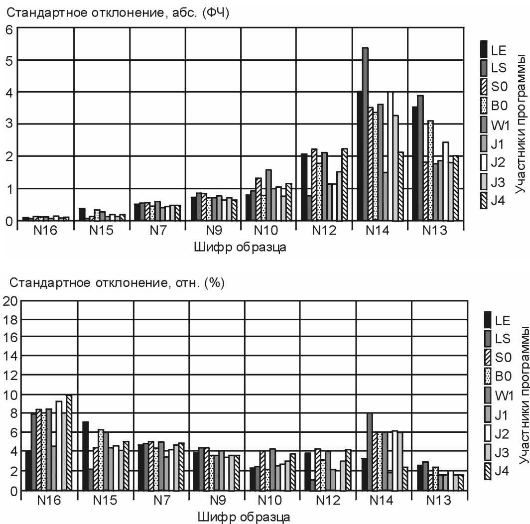
Рисунок Б.3. Результаты измерений по 6-й программе круговых сличений Раунд Робин, II Комиссия МИС - в центре рабочей стороны образца ("рабочая точка")
