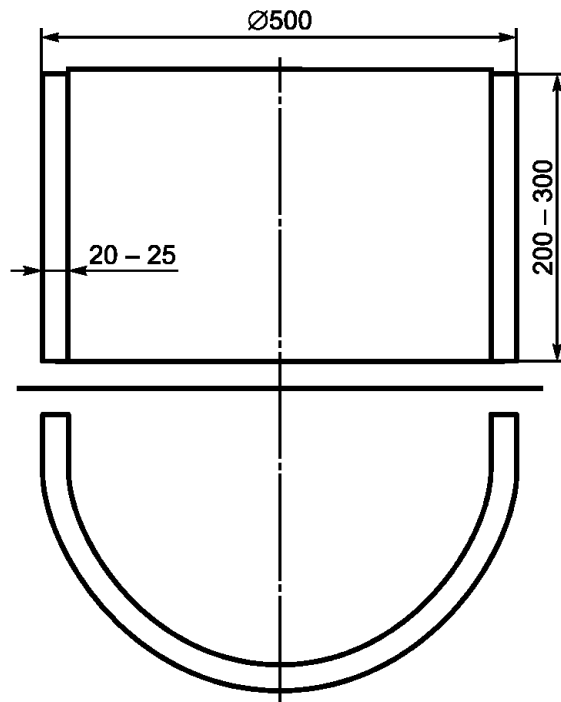
Рисунок 3. Центробежнолитая трубная заготовка для изготовления СО СФФ
