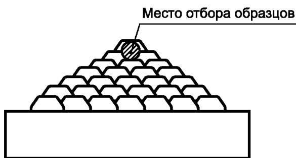
Рисунок 5. Схема выполнения семислойной наплавки покрытыми электродами и проволокой
